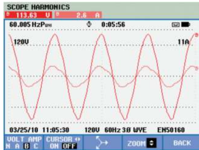
Figura 1. Carga no lineal. Observar un conjunto de ondas sinusoidales monofásicas de tensión y corriente, provocadas por una carga no lineal de distorsión muestra fácilmente que la forma de onda de la corriente (más baja) no se ajusta de ninguna manera a la forma de onda de tensión aplicada. Dichas cargas no lineales producen corrientes de armónicos que fluyen por el sistema de distribución.
