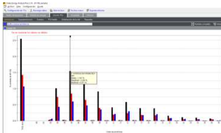
Figura 2. Armónicos. En esta pantalla de un analizador de la calidad eléctrica, las frecuencias de armónicos aparecen en el eje del armónico. El porcentaje al que se encuentra la frecuencia específica de los armónicos es un componente de la frecuencia fundamental de 50 Hz que aparece en el eje vertical. El cursor se ha colocado sobre la frecuencia del quinto armónico y la corriente de este armónico parece representar aproximadamente el 1.547% de la frecuencia de 50 Hz.
